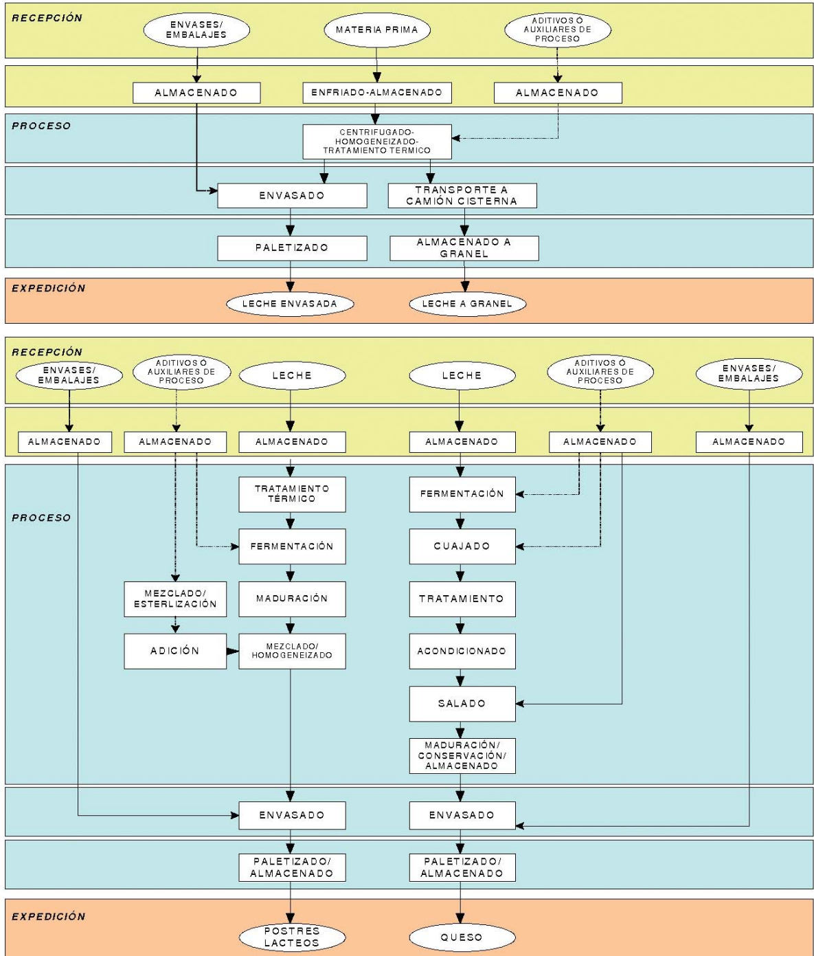
FIGURA 1. FLUJOGRAMA DEL PROCESO DE ELABORACIÓN DE LECHE, QUESO Y POSTRES LÁCTEOS
