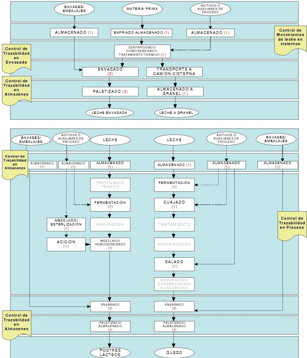
FIGURA 1: FLUJOGRAMA DE TRAZABILIDAD EN LOS PROCESOS DE ELABORACIÓN DE LECHE, QUESO Y POSTRES LACTEOS.
